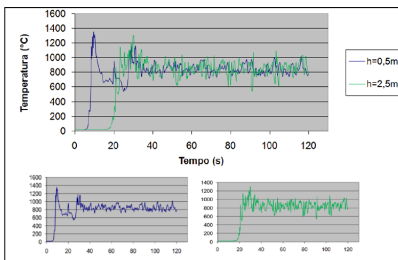
Figura 6: Temperaturas atingidas na base (esquerda) e topo (direita) do pilar P221 no segundo pavimento, interior da loja do foco do incêndio.
